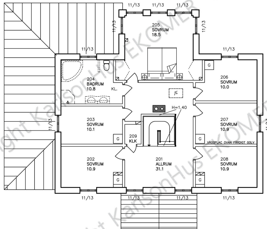
ÖVERPLAN BOA 121.4m 2
