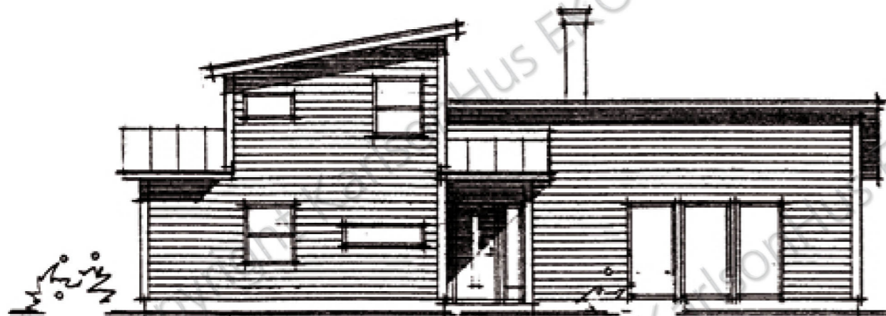
VILLA LUNDEN • FASAD MOT VÄSTER
